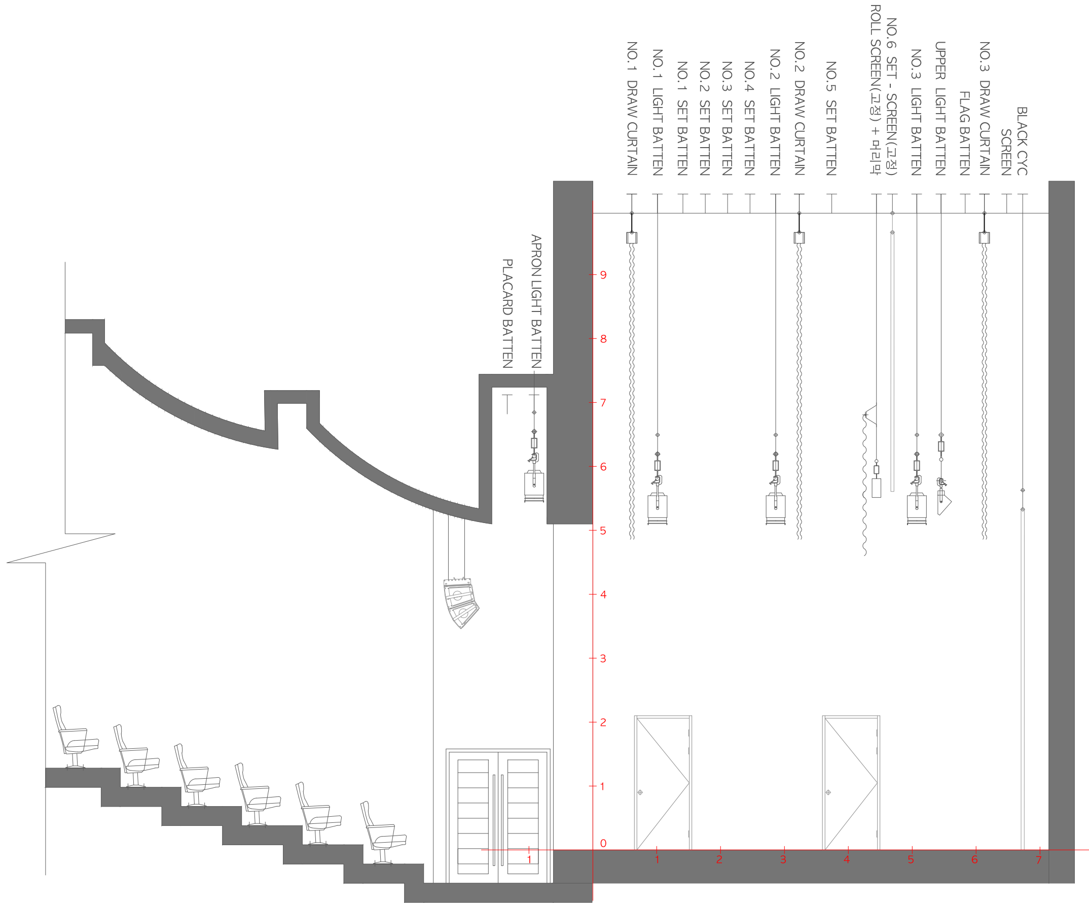
와룡홀 단면도 SCALE : 1/60
